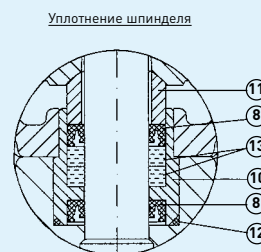
Уплотнение шпинделя
